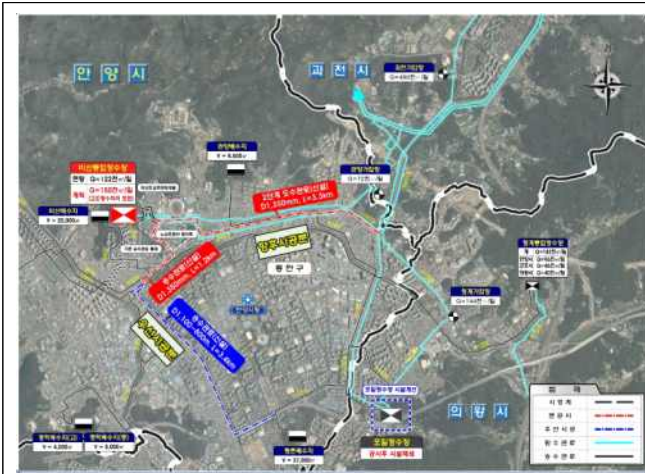
전체계획 위치도
